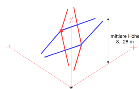
zu Bild 10: vertikal und horizontal polarisierte VDA-Antenne
