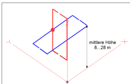
zu Bild 9: vertikal und horizontal polarisierte Moxon-Antenne
